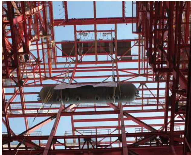
Izaje Caldera Campiche
